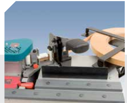
Tapesnijder en rolhouder RC50T (voor MEB250, MEB100)
