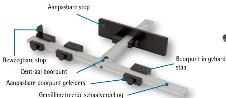
Voor het plaatsen van schappen.
