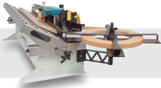
5046703 AK97NW kantentrimmer en aandrukrollen (voor MEB250 en MEB250A)
