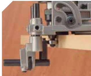
Laterale geleider vermijdt dat u onregelmatigheden kopieert.
