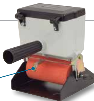
Lijmen met bovenroller
