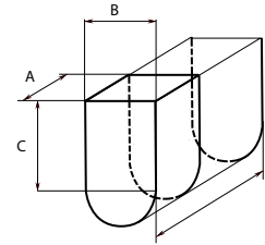
Afmeting van freesketting: b.v 28 x 40 x 100, kettingbreedte 28 mm, gatbreedte 40 mm, steekdiepte 100 mm
